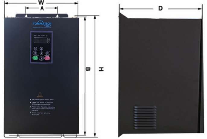
18.5KW-132KW METAL KASA
